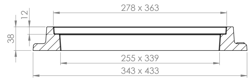
SECTION A-A SCALE 1 : 3
