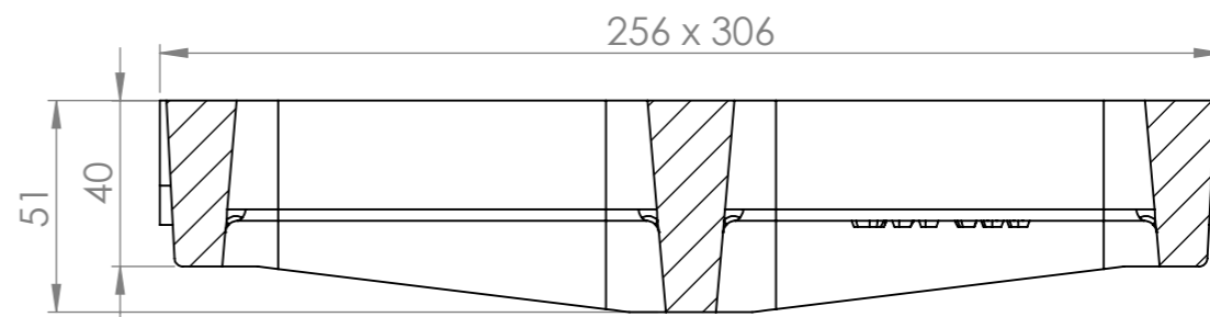
SECTION A-A
