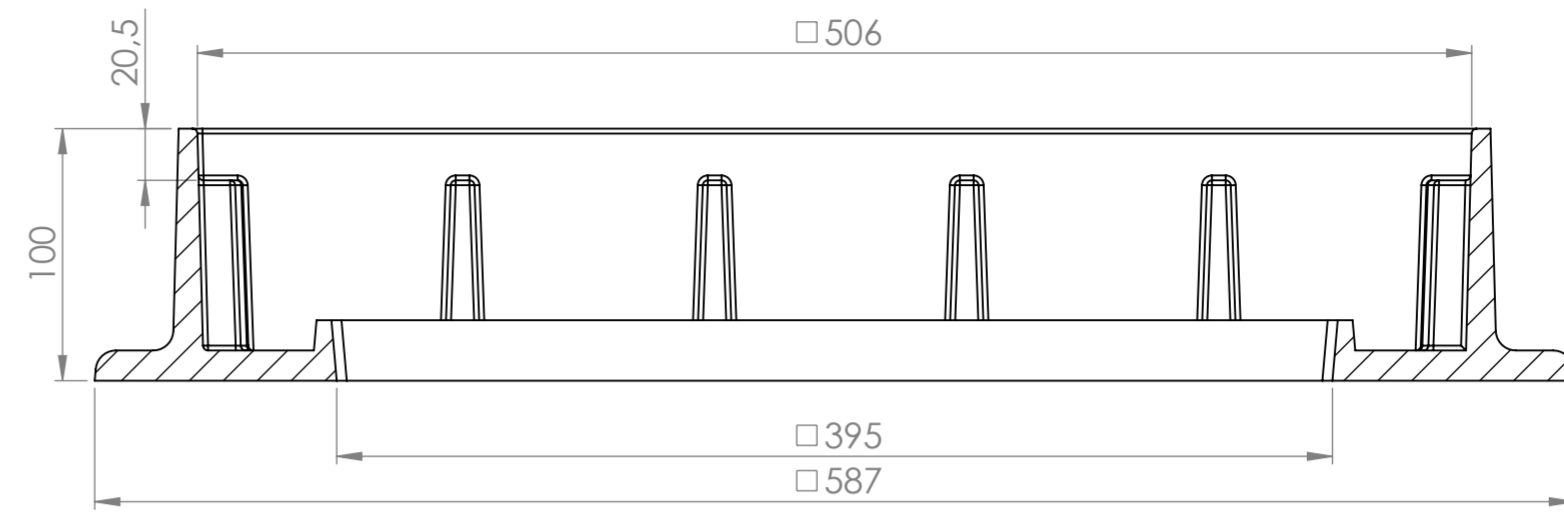
SECTION A-A SCALE 1 : 3
