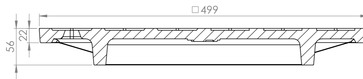
SECTION A-A
