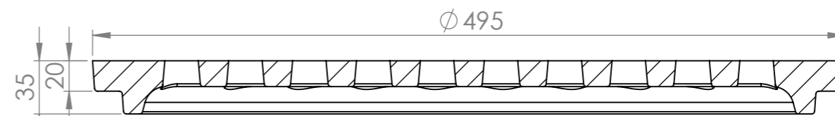
SECTION A-A
