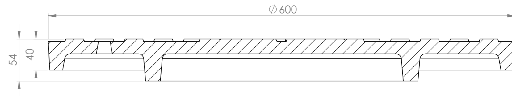
SECTION A-A
