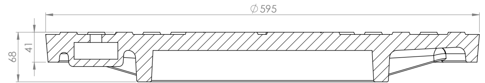
SECTION A-A
