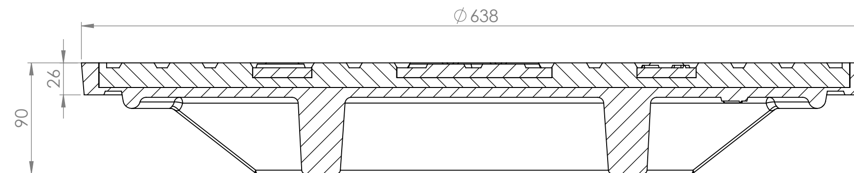
SECTION A-A SCALE 1 : 3
