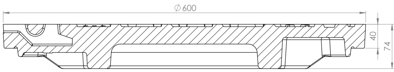
SECTION A-A SCALE 1 : 4
