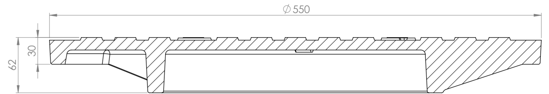
SECTION A-A
