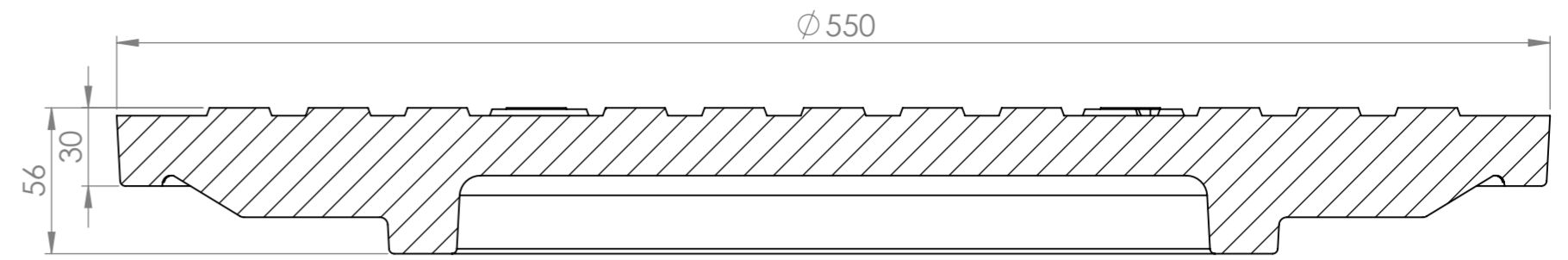
SECTION A-A
