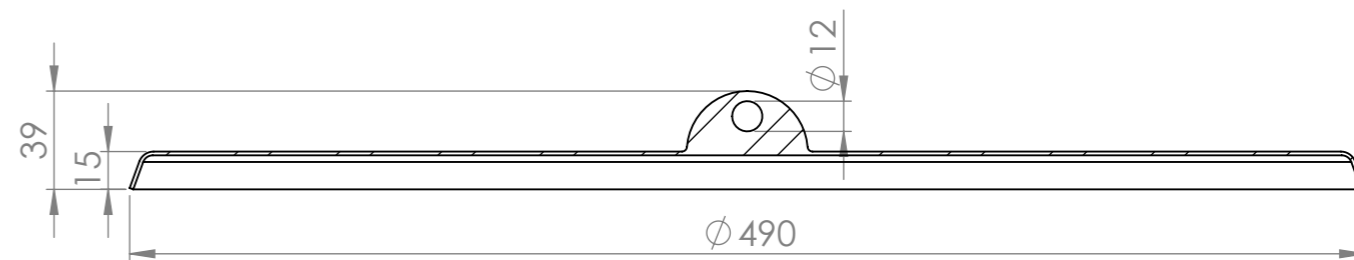
SECTION A-A
