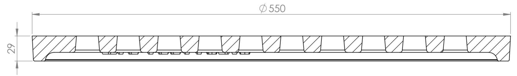
SECTION A-A
