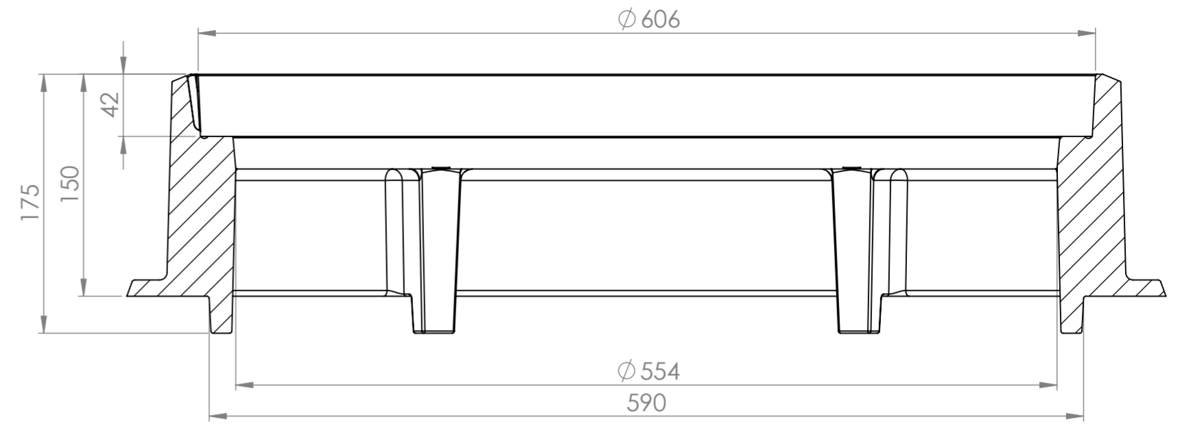
SECTION A-A
