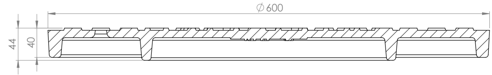
SECTION A-A
