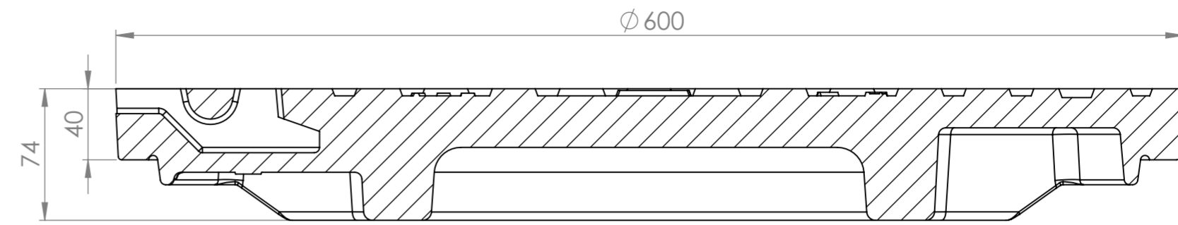
SECTION A-A
