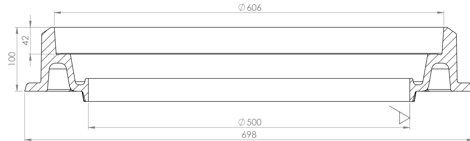
SECTION A-A
