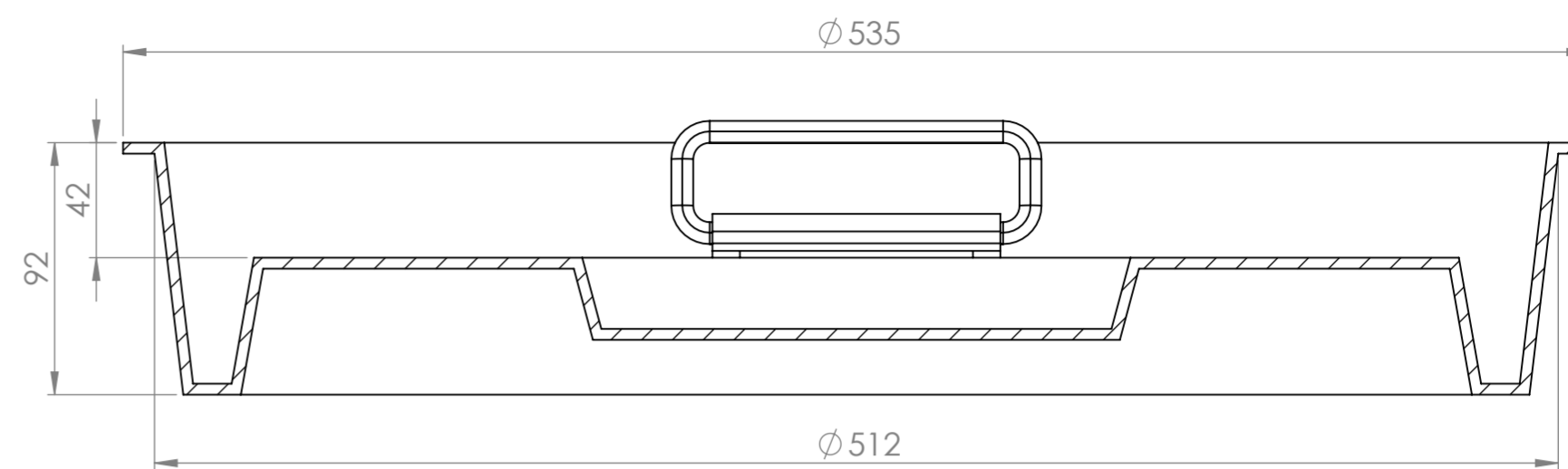
SECTION A-A
