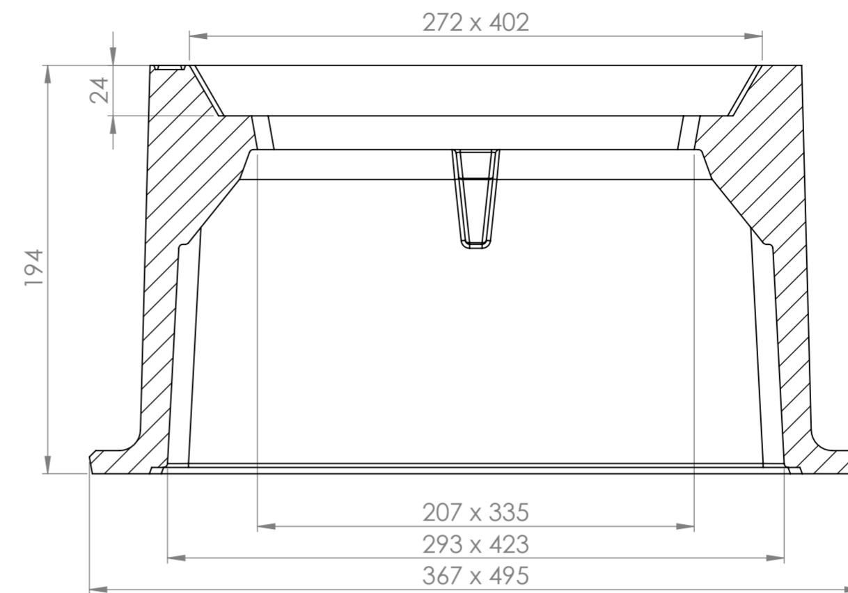
SECTION A-A
