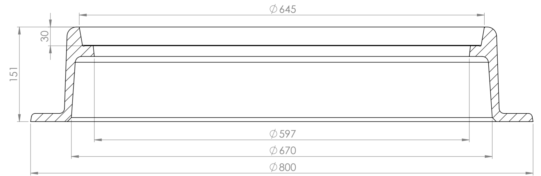
SECTION A-A
