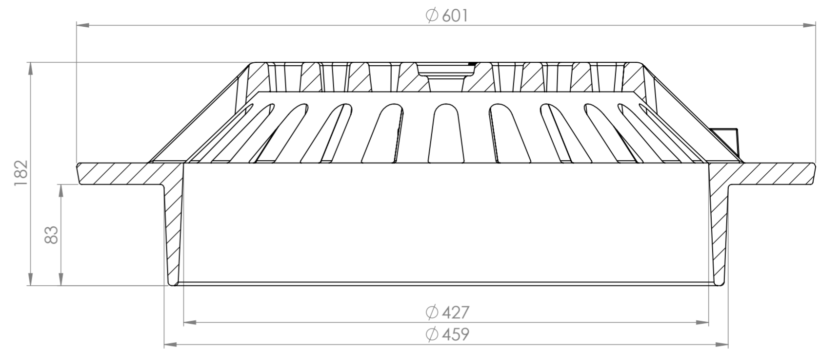
SECTION A-A
