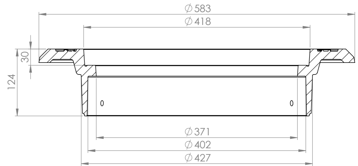
SECTION A-A
