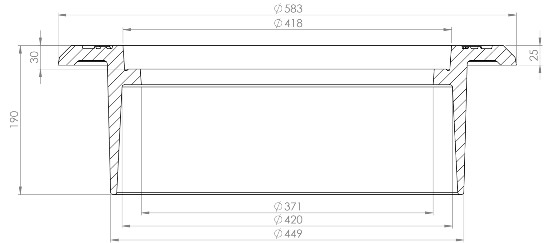
SECTION A-A SCALE 1 : 3
