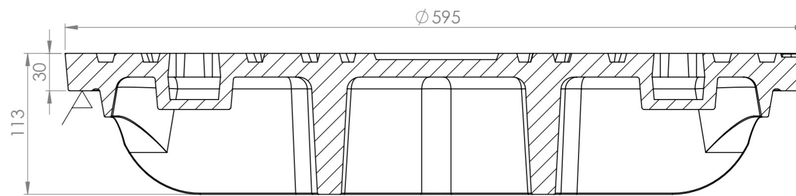
SECTION A-A
