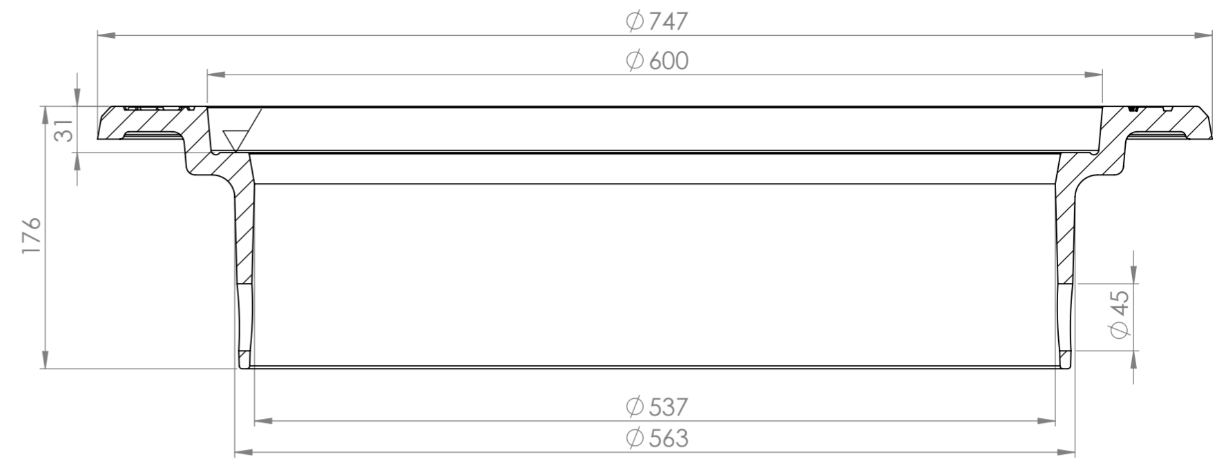
SECTION A-A
