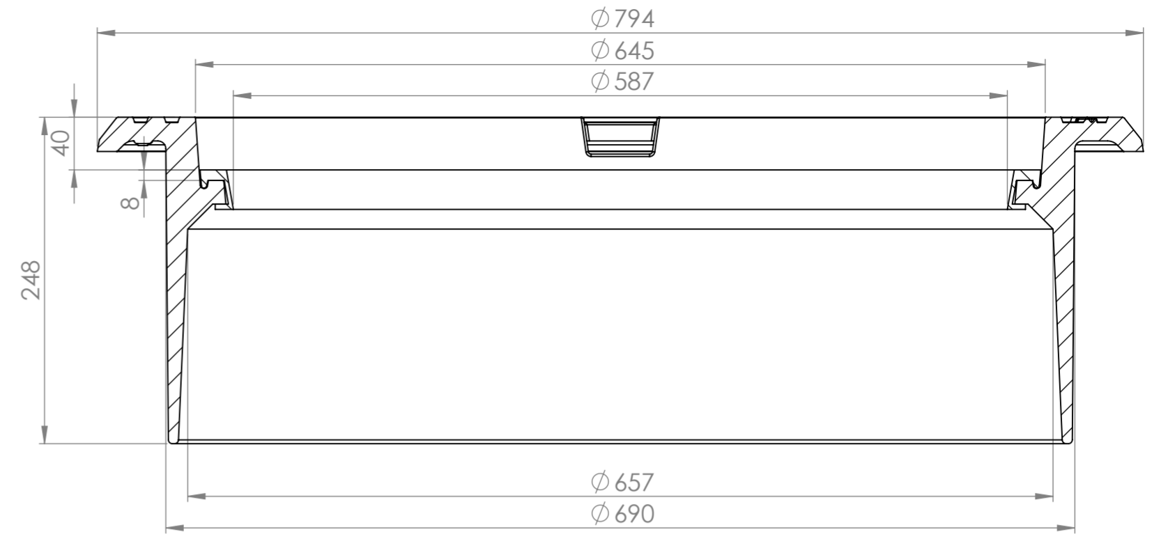
SECTION A-A
