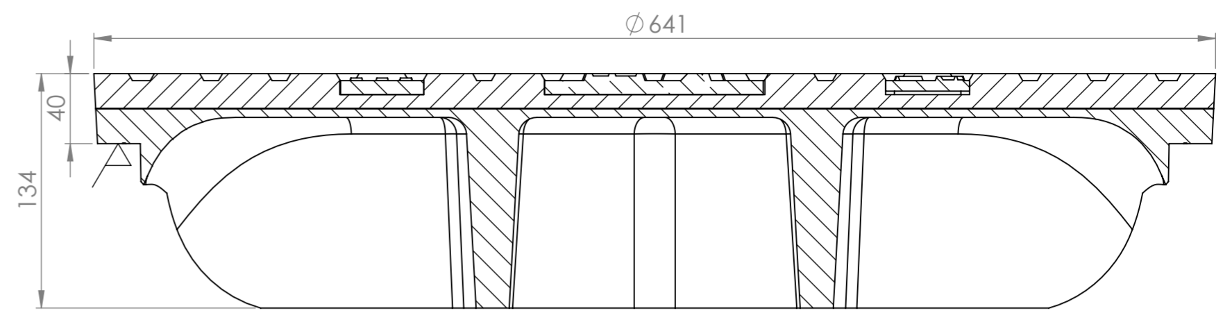
SECTION A-A
