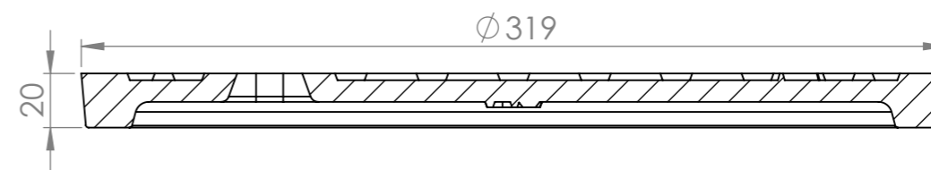
SECTION A-A
