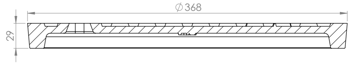
SECTION A-A
