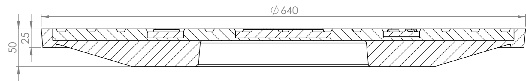
SECTION A-A
