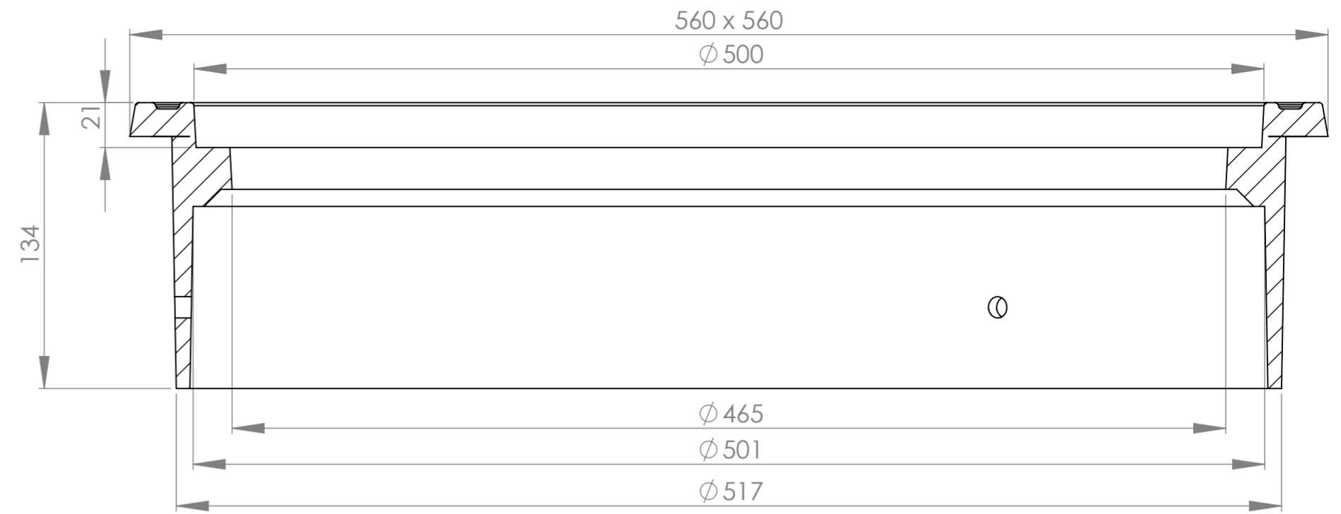
SECTION A-A
