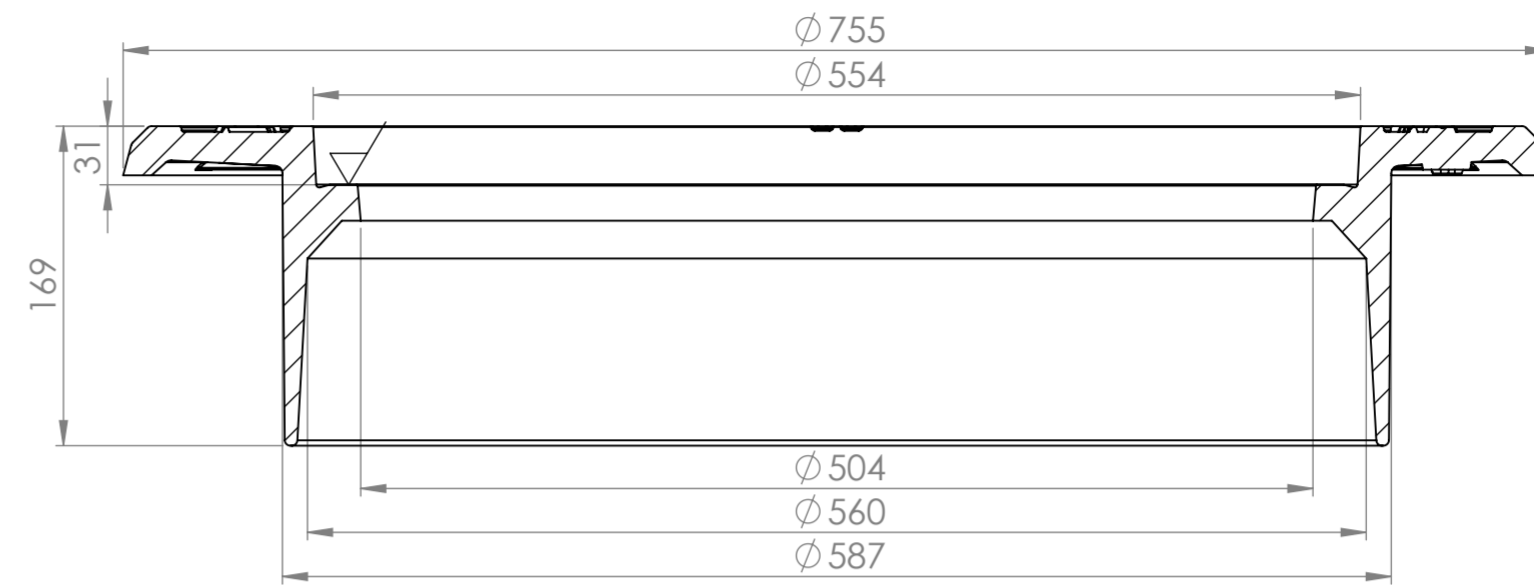
SECTION A-A
