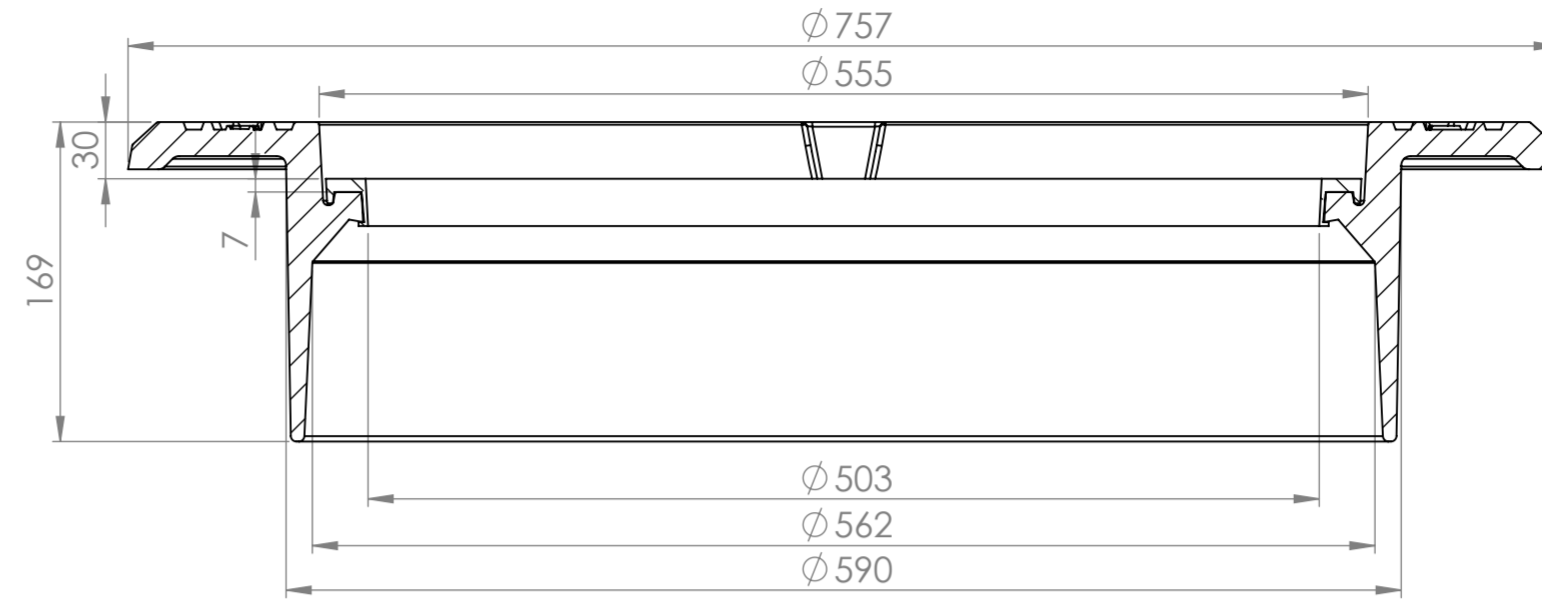
SECTION A-A
